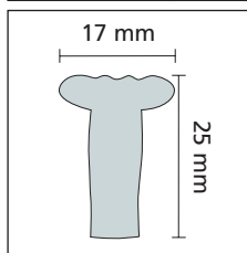
Sezione griglia tipo perpendicolare Coupe des grilles perpendiculaires Section of perpendicular gratings Schnitt des rechtwinklige Abdeckroste
