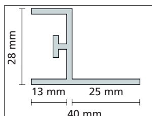
Sezione supporto griglia in PVC Coupe support des grilles en PVC Section of gratings support Schnitt des rostträgers aus PVC
