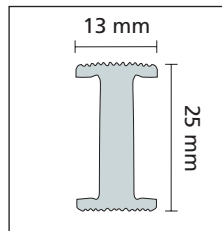
Sezione griglia tipo parallelo Coupe des grilles paralleles Section of parallel gratings Schnitt des parallele Abdeckrostes
