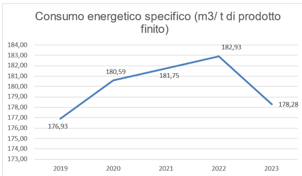
Figura 29 - Andamento del consumo energetico specifico per tonnellata di prodotto finito (Sm 3 /t)
