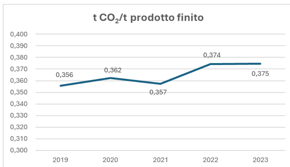
Figura 36 - Produzione di anidride carbonica per unità di peso (tCO 2 /t)
