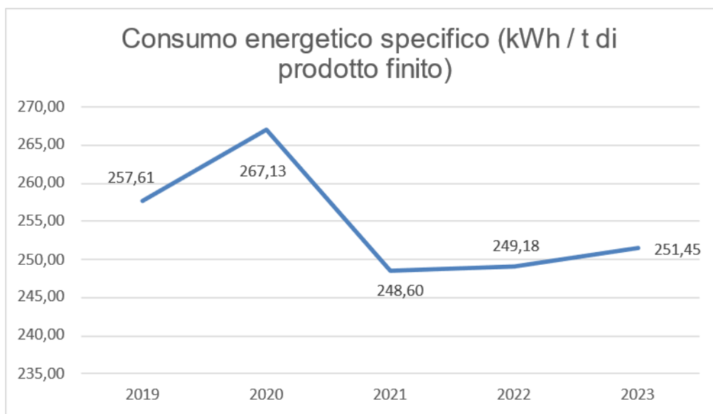
Figura 26 - Consumo energetico specifico (kWh/tonnellate di prodotto finito)
