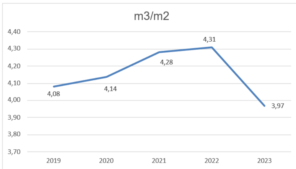
Figura 28 - Andamento del consumo specifico di metano per unità di prodotto ( \text{Sm}^3/\text{m}^2 )
