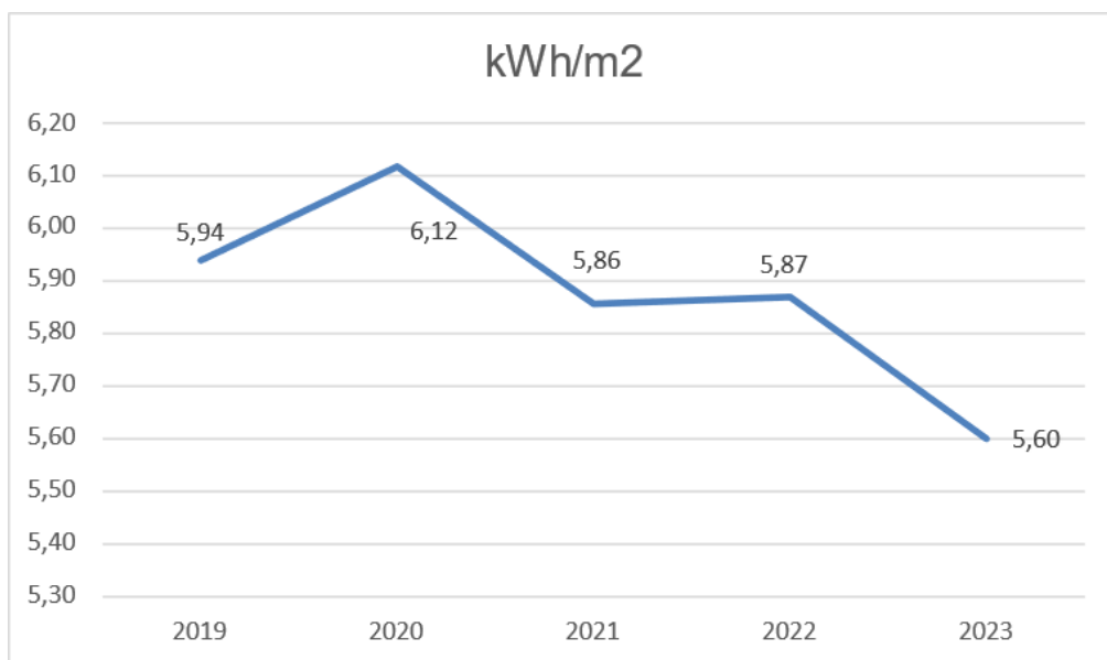
Figura 25 - Consumo energetico specifico (kWh/m 2 finito)
