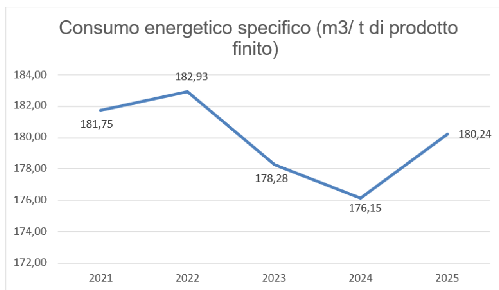
Figura 33 - Andamento del consumo energetico specifico per tonnellata di prodotto finito (Sm 3 /t)
