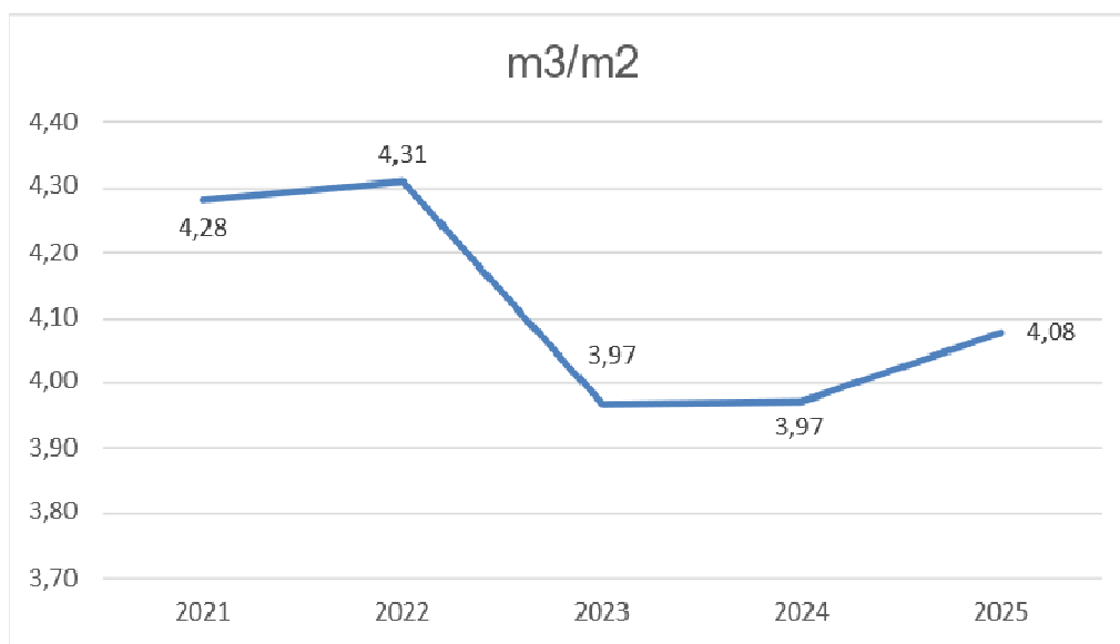
Figura 32 - Andamento del consumo specifico di metano per unità di prodotto (Sm 3 /m 2 )
