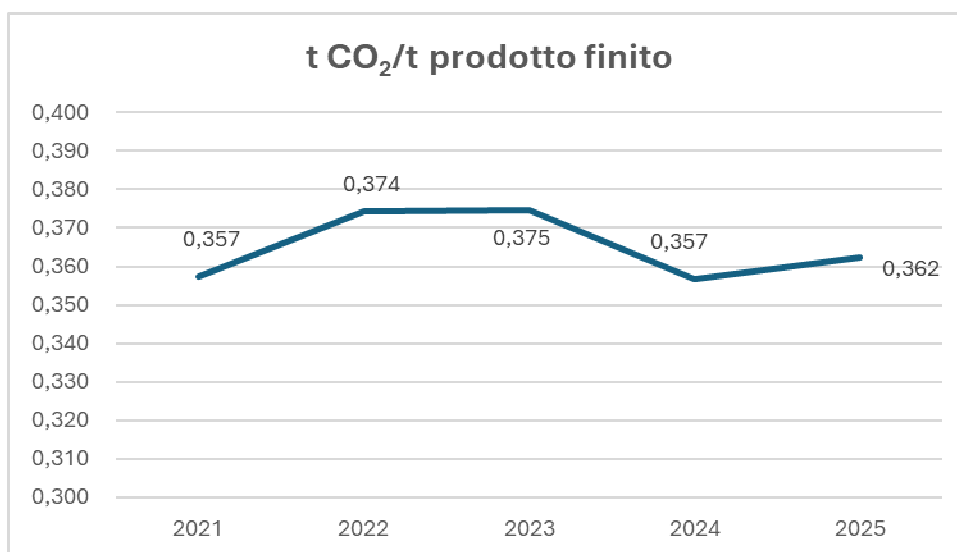
Figura 40 - Produzione di anidride carbonica per unità di peso (tCO 2 /t)
