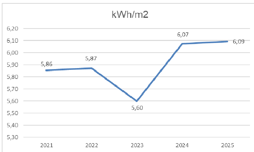
Figura 29 - Consumo energetico specifico (kWh/m² finito)
