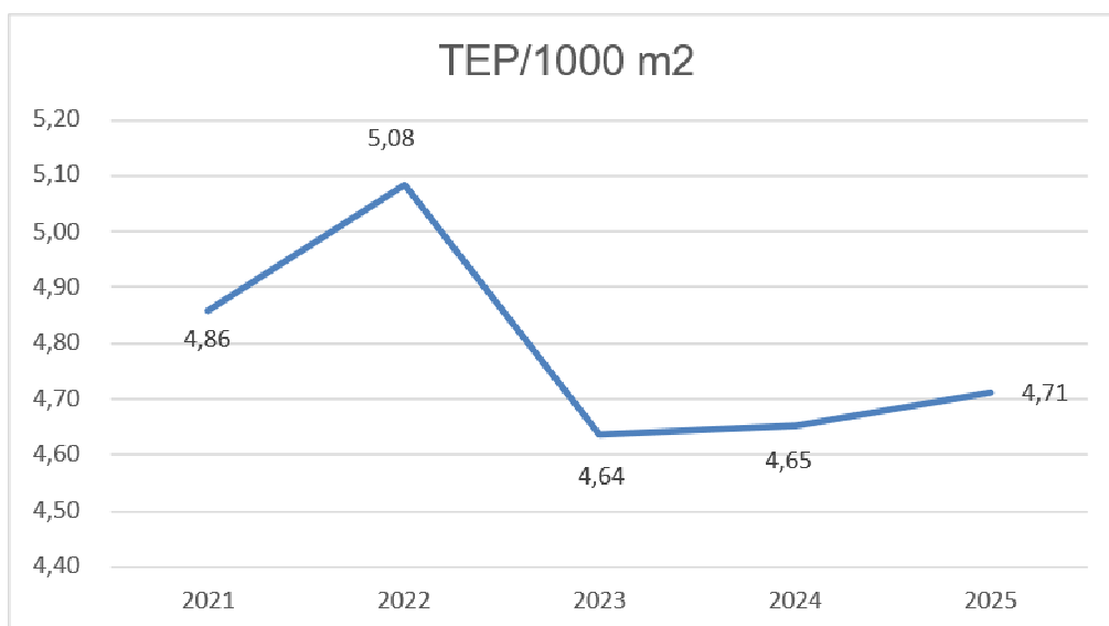
Figura 36 - Consumo energetico su tonnellata di prodotto finito (TEP/1000 m 2 )
